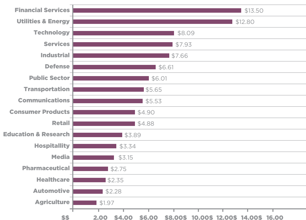
Figura 3 – Custo médio atualizado por setor de indústria (milhões). Reproduzido de The cost of incidents affecting CIIs.
